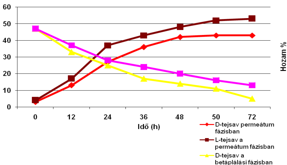
1. ábra A tejsav enantiomerjei koncentrációinak változása ionos folyadék (Cyphos 104) folyadékmembrán alkalmazásával, a kísérleti idő függvényében.
