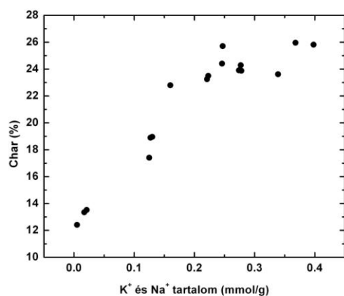
1. ábra: Összefüggés a kender hőbomlási paramétereinek valamint a nátrium és kálium-tartalom mennyisége között lúggal különbözőképpen kezelt, forró vízzel mosott és kezeletlen mintákon
