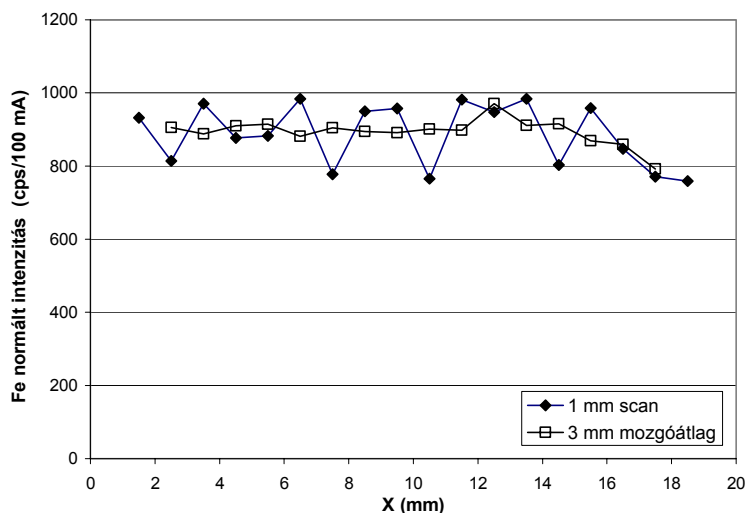
3. ábra: Az impaktált aeroszolcsík homogenitásának ellenőrzése SR-TXRF méréssel.
