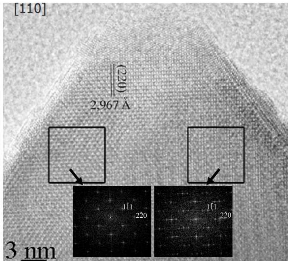
10. ábra. Doménes szerkezetű maghemit kristály, a bekeretezett részekről készült Fourier transzformokkal. A jobb oldali területen látszik a superperiodicitás, utalva a vakancia-rendezett, tetragonális változatra, míg a bal oldalon a szerkezet köbös.
