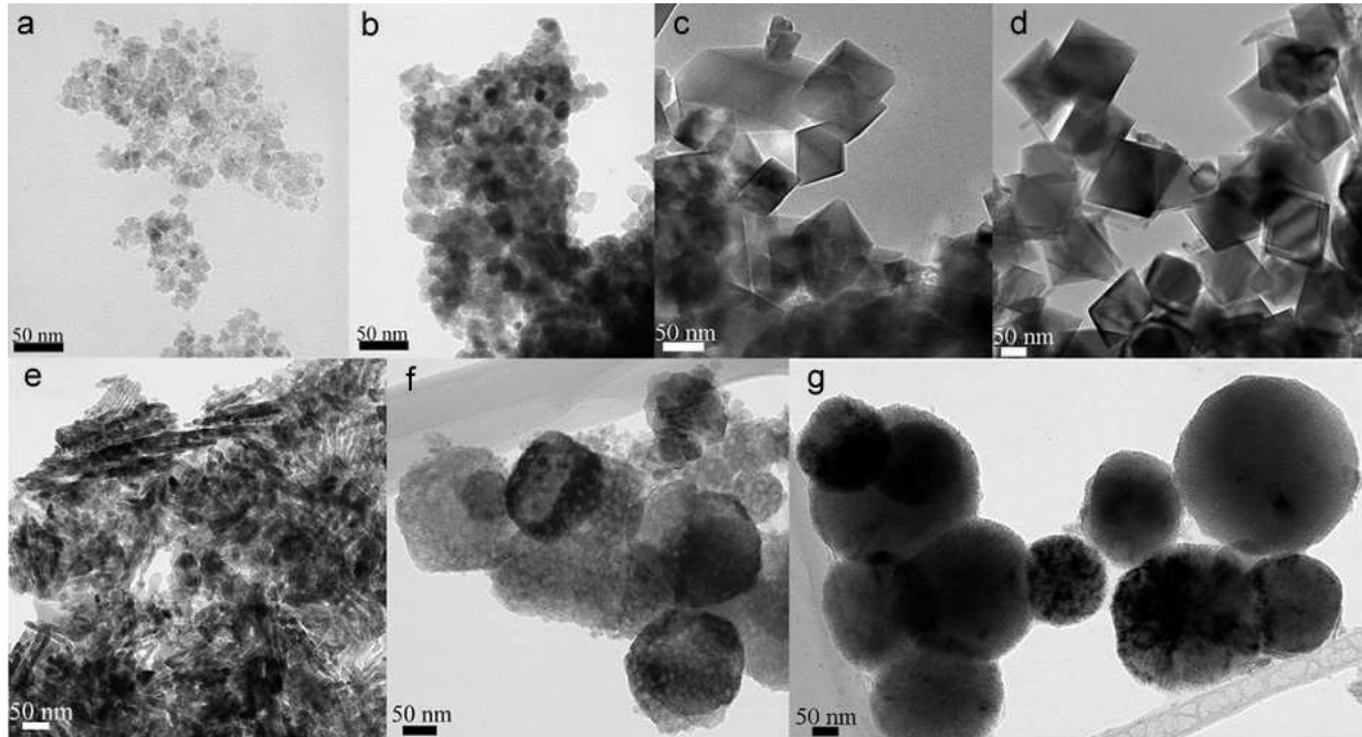
7. ábra. Változatos morfológiájú, szintetikus magnetit nanokristályok. (a) Szabálytalan; (b) kerekded; (c, d) oktaéderez; (e) megnyúlt, léces kristályok. (f) Heterogén kontrasztú aggregátumok. (g) Korong alakú aggregátumok.
