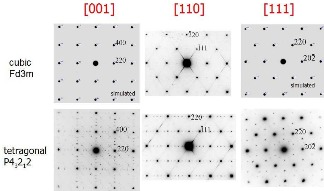
9. ábra. Maghemit kristályokról készült elektrondiffrakciós felvételek három különböző vetületben. A felső sor köbös, az alsó tetragonális szimmetriájú, vakancia-rendezett változatról készült. A tetragonális változatról készült felvételeken jól láthatók a szupercella reflexiók.
