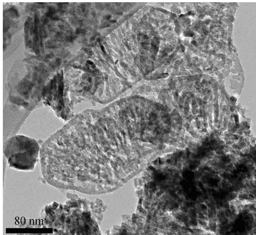
8. ábra. Szulfát zöld rozsda közttermékből képződött magnetit kristályok, amelyek őrzik az elődfázis hexagonális morfológiáját.
