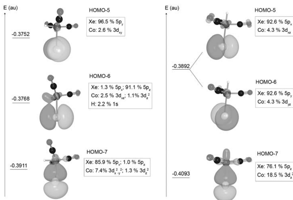
2. ábra. A C_s és C_{3v} szimmetriájú \text{HCo(CO)}_3\text{Xe} adduktok természetes populáció analízis segítségével kapott kölcsönható kanonikus orbitáljai.
